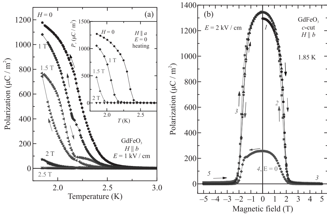
Рис. 3. (Цветной онлайн) (а) – Температурные зависимости поляризации вдоль оси c в разных магнитных полях H \parallel b . Стрелки показывают направление изменения температуры (охлаждение или нагрев). На вставке зависимость P_c(T) при нагреве в E = 0 в разных H \parallel a . (б) – Зависимость поляризации от магнитного поля H \parallel b при T = 1.85 К. Номера у кривых – последовательность сканирования по полю (1 – 0 → 5 Тл; 2 – 5 Тл → –5 Тл; 3 – –5 Тл → 5 Тл; 4 – 5 Тл → –5 Тл; 5 – –5 Тл → 0). Кривые 1, 2, 3 и 5 измерены в E = 2 кВ/см, кривая 4 – в E = 0
