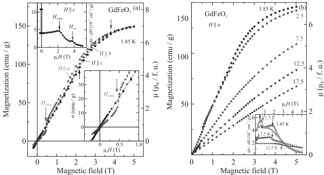
Рис. 2. (Цветной онлайн) Кривые намагничивания: (а) – вдоль осей a , b и c при T = 1.85 \text{ K} ; на нижней вставке – в увеличенном масштабе, на верхней – производная d\sigma/dH_c . Стрелками отмечены фазовые переходы: красной – спин-флоп при H \parallel a , черной – спин-флип и темно-зеленой – переворот спонтанного момента железа вдоль поля при H \parallel c (всплески d\sigma/dH_c в полях \sim \pm 1 \text{ кЭ} вызваны переворотом результирующего момента Gd и Fe подсистем). (б) – Вдоль a -оси при разных температурах. На вставке – производные d\sigma/dH_a . Стрелками отмечены поля фазовых переходов
