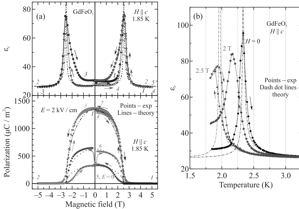
Рис. 4. (Цветной онлайн) (а) – Зависимость поляризации P_c (нижняя панель) и диэлектрической проницаемости \epsilon_c (верхняя панель) от магнитного поля H \parallel c при T = 1.85 К. Номера у кривых P_c показывают последовательность сканирования по полю (1 – 0 → 5 Тл; 2 – 5 Тл → –5 Тл; 3 – –5 Тл → 0; 4 – 0 → 5 Тл; 5 – 5 Тл → –5 Тл; 6 – –5 Тл → 5 Тл; 7 – 5 Тл → 0). Кривые 1, 2, 3 и 7 измерены в E = 2 кВ/см, кривые 4, 5 и 6 – в E = 0 . Аналогично для \epsilon_c кривая 1 соответствует 0 → 5 Тл; 2 – 5 Тл → –5 Тл; 3 – –5 Тл → 0; 4 – 0 → 5 Тл; 5 – 5 Тл → 0. Точки – эксперимент; пунктирные и штрихпунктирные линии – теория. (б) – Температурные зависимости \epsilon_c в разных магнитных полях H \parallel c . Точки – эксперимент; штрихпунктирные линии – теория. Стрелки показывают направление изменения температуры
