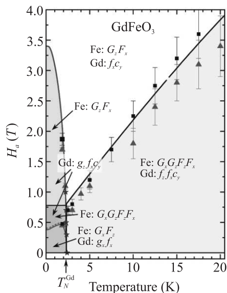
Рис. 6. (Цветной онлайн) Фазовая диаграмма \text{GdFeO}_3 при H \parallel a . Точки – эксперимент: черные квадраты – \sigma(H) , красные треугольники – из \varepsilon(H) , синие звездочки – из \varepsilon(T) . Линии – теория: синяя разделяет угловую магнитную структуру \Gamma_{24} и индуцированную слабоферромагнитную структуру \Gamma_2 (полное описание структур через векторы антиферро- и ферромагнетизма приведены на рисунке). Зеленая линия отражает спин-флип переход Gd, черная горизонтальная линия разделяет фазы \Gamma_{24} и \Gamma_2 железа, фиолетовая – линия спин-флоп перехода Gd ( H_{x1} ), красная пунктирная – расчетная линия ( H_{x2} ) для случая одновременной спиновой переориентации Gd и Fe подсистем (см. текст)
