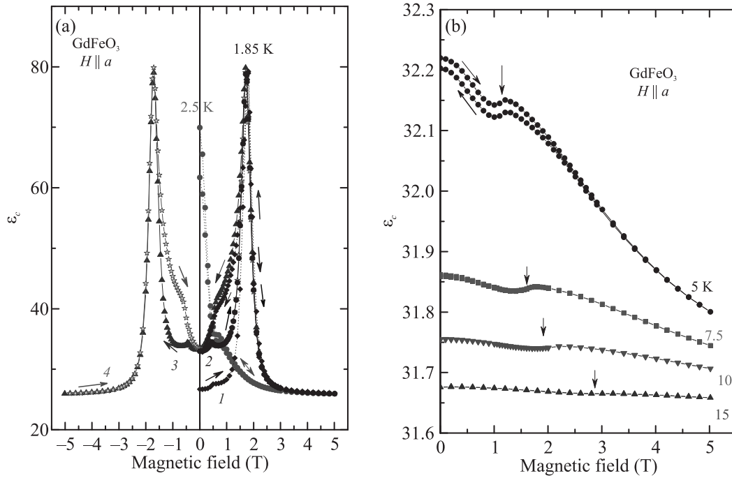
Рис. 5. (Цветной онлайн) Зависимость диэлектрической проницаемости от магнитного поля H \parallel a : (a) – при T = 1.85 K (кривая 1 измерена после поляризации образца в электрическом поле E = 2 кВ/см, а остальные кривые 2 – 4 в E = 0 ) и T = 2.5 K. Номера показывают последовательность сканирования по полю (1 – 0 \rightarrow 5 Тл \rightarrow 0 ; 2 – 0 \rightarrow 5 Тл; 3 – 5 Тл \rightarrow -5 Тл; 4 – -5 Тл \rightarrow 5 Тл). (b) – При температурах выше T_N^{\text{Gd}} . Стрелками отмечены аномалии на кривых \varepsilon_c(H_a)
