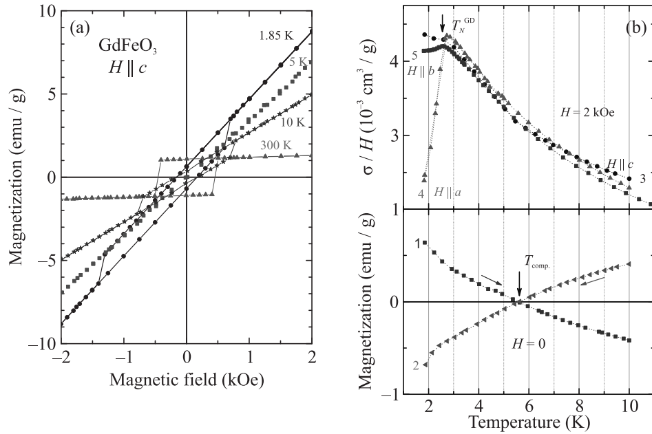
Рис. 1. (Цветной онлайн) (а) – Кривые намагничивания \text{GdFeO}_3 вдоль оси c при разных температурах. (б) – Температурные зависимости остаточной намагниченности вдоль оси c (нижняя панель) после предварительного намагничивания при T = 1.9 \text{ K} (кривая 1) и при T = 10 \text{ K} (кривая 2) и DC восприимчивости \sigma/H (верхняя панель) в H \parallel c – кривая 3, H \parallel a – кривая 4 и H \parallel b – кривая 5)
