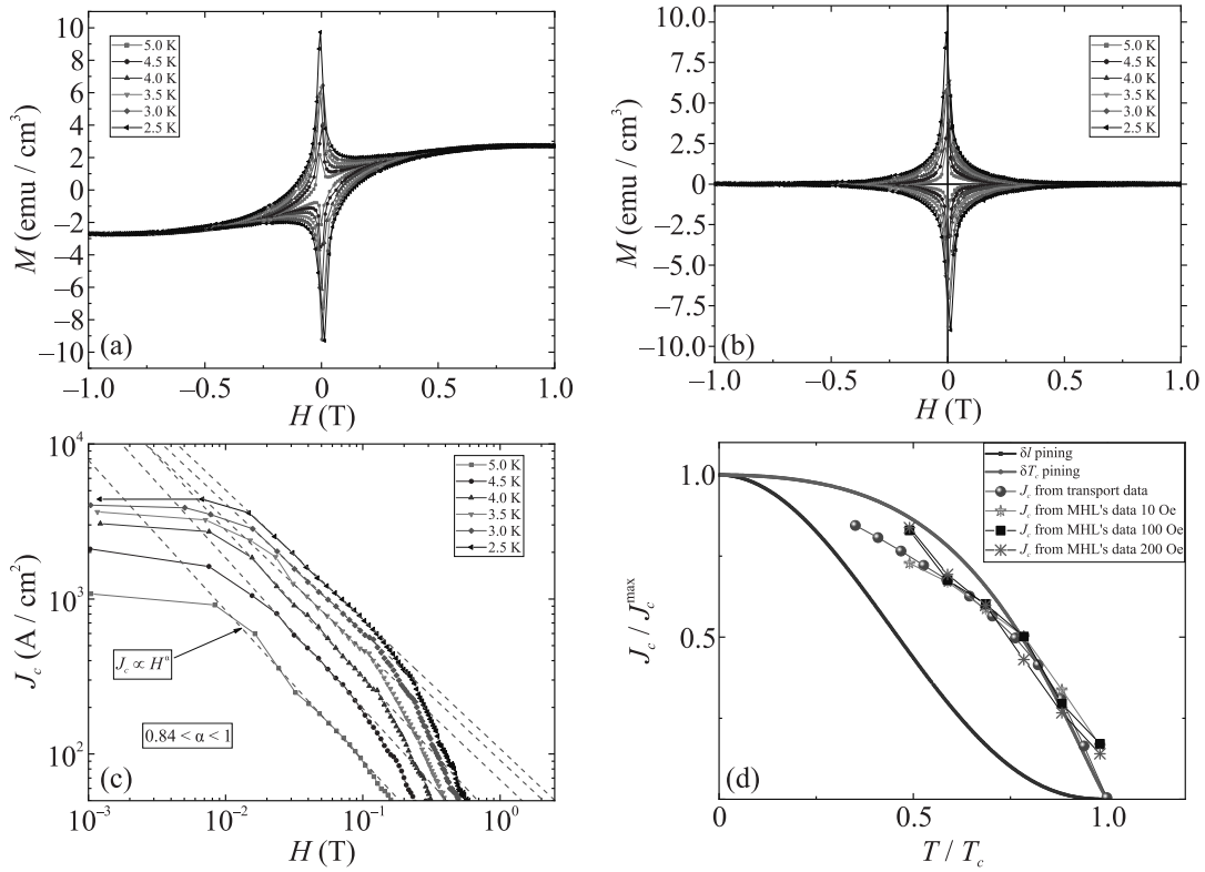
Рис. 2. (Цветной онлайн) Зависимость магнитной восприимчивости от внешнего поля при различных температурах до (a) и после (b) вычитания парамагнитного вклада. (c) – Моделирование критической плотности тока по модели Бина. (d) – Нормированные значения плотности тока, модельные кривые l и T_c обозначены черной и красной линиями соответственно
