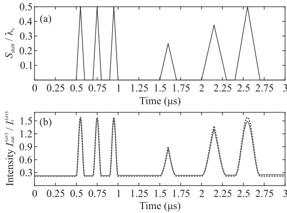
Рис. 2. (Цветной онлайн) Временная зависимость: (а) – функции смещения источника ^{67}\text{Ga} или ^{67}\text{Cu} (13), (14) для M = 6 и (б) – соответствующей нормированной интенсивности потока фотонов с энергией 93.3 кэВ на выходе из резонансного поглотителя ^{67}\text{ZnS} в случае T_a = 3.2 ( L = 2.56 мм) и T_e = 0.15T_a . Для функции смещения (13), (14) t_{\text{start}}^{(1)} = 0.5 мкс, t_{\text{start}}^{(2)} = 0.7 мкс, t_{\text{start}}^{(3)} = 0.9 мкс, t_{\text{start}}^{(4)} = 1.5 мкс, t_{\text{start}}^{(5)} = 2 мкс, t_{\text{start}}^{(6)} = 2.4 мкс, \Delta t_b^{(i)} = \Delta t_f^{(i)} = 0.05 мкс ( i = 1, 2, 3 ), \Delta t_b^{(4)} = \Delta t_f^{(4)} = 0.1 мкс, \Delta t_b^{(i)} = \Delta t_f^{(i)} = 0.15 мкс ( i = 5, 6 ), \Delta t_c^{(i)} = 0 ( i = 1, \dots, 6 ), \Delta z^{(i)} = \lambda_s/2 ( i = 1, 2, 3, 6 ), \Delta z^{(4)} = \lambda_s/4 , \Delta z^{(5)} = 3\lambda_s/8 . Зеленые пунктирные и красные сплошные линии построены с использованием выражений (12) и (8)–(10) соответственно
