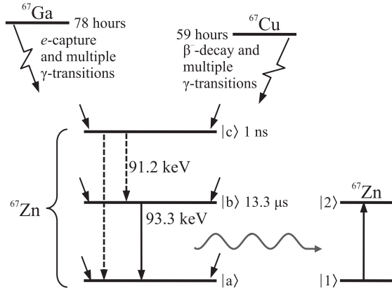
Рис. 1. (Цветной онлайн) Схема радиоактивного распада источников ^{67}\text{Ga} и ^{67}\text{Cu} (слева) и резонансного поглощения фотонов с энергией 93.3 кэВ ядром поглотителя ^{67}\text{Zn} (справа). Ядро ^{67}\text{Ga} распадается (наклонные стрелки) в результате захвата электрона, превращаясь в ядро ^{67}\text{Zn} в пяти энергетических состояниях, включая основное состояние [22]. Ядро ^{67}\text{Cu} претерпевает \beta^- -распад, превращаясь в ядро ^{67}\text{Zn} в четырех энергетических состояниях (наклонные стрелки), включая основное состояние [20, 21]. В рассматриваемом случае важны только основное и два возбужденных состояния. Возбужденные состояния ядра ^{67}\text{Zn} затем излучательно распадаются до состояний с более низкой энергией (вертикальные стрелки). Как для ^{67}\text{Ga} , так и для ^{67}\text{Cu} вероятности распада в состояние |b\rangle и в состояние |c\rangle являются величинами одного порядка [20–22]. Поэтому существенная часть фотонов с энергией 93.3 кэВ, испускаемых при переходе |b\rangle \rightarrow |a\rangle , не коррелирует с фотонами с энергией 91.2 кэВ, испускаемыми при переходе |c\rangle \rightarrow |b\rangle
