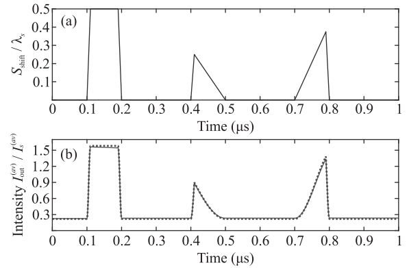
Рис. 3. (Цветной онлайн) Временная зависимость: (а) – функции смещения источника ^{67}\text{Ga} или ^{67}\text{Cu} , S_{\text{shift}}(t) , (13), (14) для M = 3 и (б) – соответствующей нормированной интенсивности потока фотонов с энергией 93.3 кэВ на выходе из резонансного поглотителя ^{67}\text{ZnS} в случае T_a = 3.2 ( L = 2.56 мм) и T_e = 0.15T_a . Для функции смещения (13), (14), t_{\text{start}}^{(1)} = 0.1 мкс, \Delta t_f^{(1)} = 0.01 мкс, \Delta t_c^{(1)} = 0.08 мкс, \Delta t_b^{(1)} = 0.01 мкс, \Delta z^{(1)} = \lambda_s/2 , t_{\text{start}}^{(2)} = 0.4 мкс, \Delta t_f^{(2)} = 0.01 мкс, \Delta t_c^{(2)} = 0 , \Delta t_b^{(2)} = 0.09 мкс, \Delta z^{(2)} = \lambda_s/4 , t_{\text{start}}^{(3)} = 0.7 мкс, \Delta t_f^{(3)} = 0.09 мкс, \Delta t_c^{(3)} = 0 , \Delta t_b^{(3)} = 0.01 мкс, \Delta z^{(3)} = 3\lambda_s/8 . Зеленые пунктирные и красные сплошные линии построены с использованием выражений (12) и (8)–(10) соответственно
